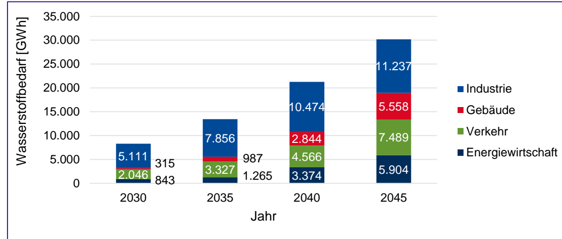
Hochlauf und Zusammensetzung der Wasserstoffbedarfsprognose bis 2045 – Szenario „Hessen“
