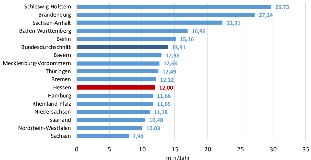
Abbildung 47: Versorgungsunterbrechungen (SAIDI) Strom nach Bundesländern 2018 (in min/Jahr)
