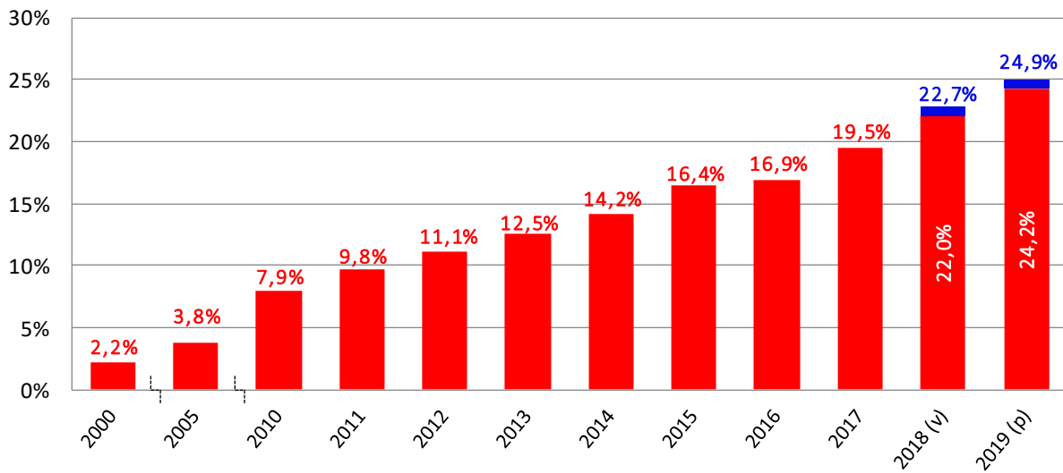
Abbildung 25: Anteilentwicklung erneuerbarer Energien am Bruttostromverbrauch 2000-2019* (in %)
