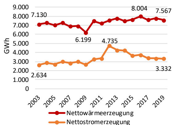
Abbildung 40: Entwicklung der Nettostrom- und Nettowärmeerzeugung durch KWK-Anlagen 2003-2019 (in GWh*)
