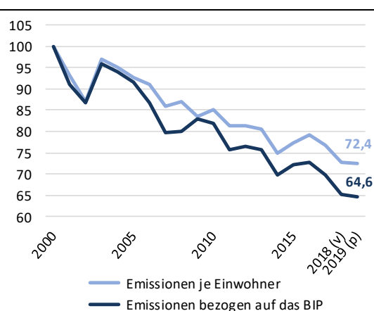
Abbildung 58: Entwicklung der Treibhausgasemissionen je Einwohner und bzgl. BIP* (Index 2000 = 100)
